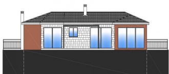
SJEVERNO PROČELJE 1:100
